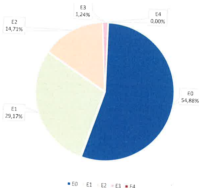
Slika 5 Bilanca pokrivenosti zona rasvijetljenosti
