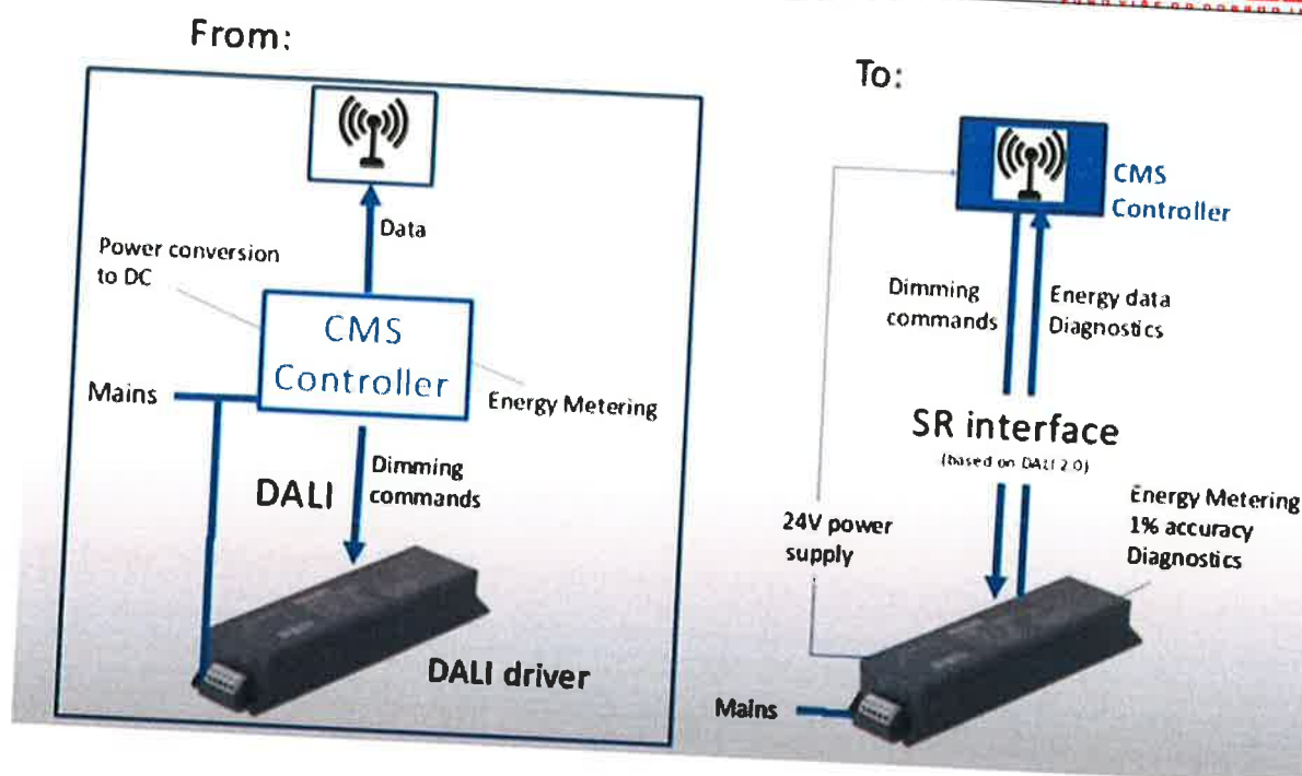
Slika 8 Prednosti SR drivera za sustav upravljanja
